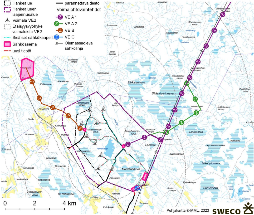
Kuva 3 Voimalasijoittelu vaihtoehdossa VE2 ja hankkeen sähkösiirtovaihtoehdot. Huom. että vaihtoehdot SVEA1 ja SVEA2 on jätetty pois suunnittelusta joulukuussa 2023.
