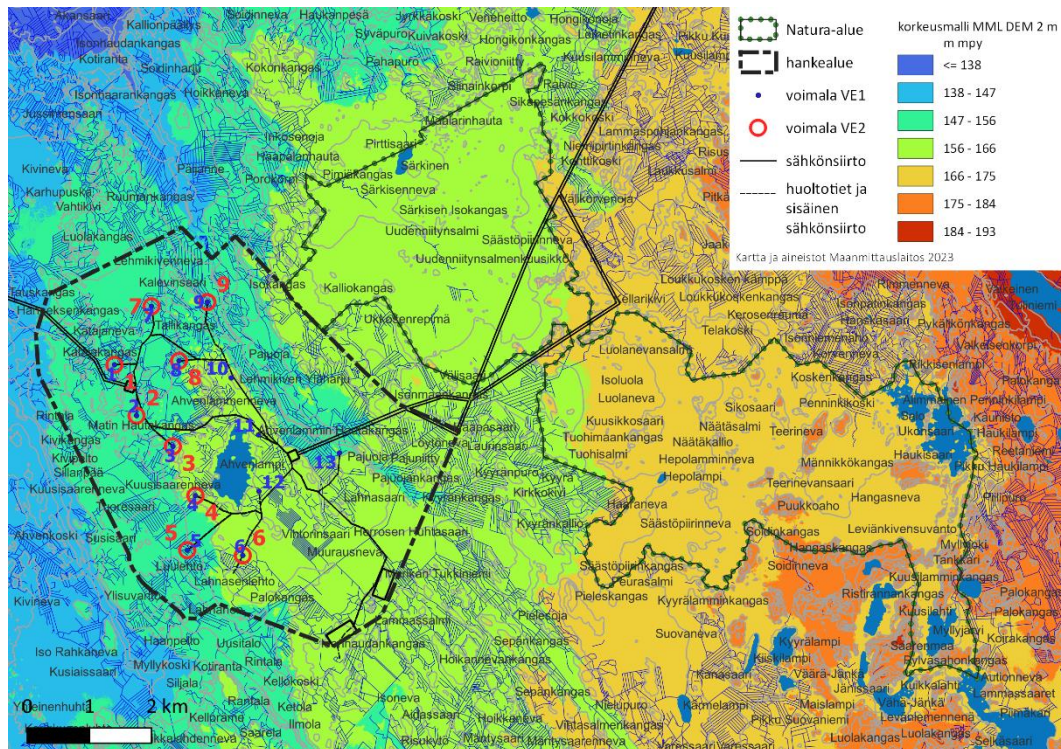
Kuva 7. Hankealueen korkeusmalli, korkeuskäyrät ja ojat Maanmittauslaitoksen aineiston mukaan. Hankevaihtoehdon VE1 voimalat on kuvassa esitetty sinisellä ja VE2 punaisella värillä. Huom. että voimalavaihto VE1 ja sähkösiirron vaihtoehdot SVEA1 ja SVEA2 on jätetty pois suunnittelusta joulukuussa 2023.
